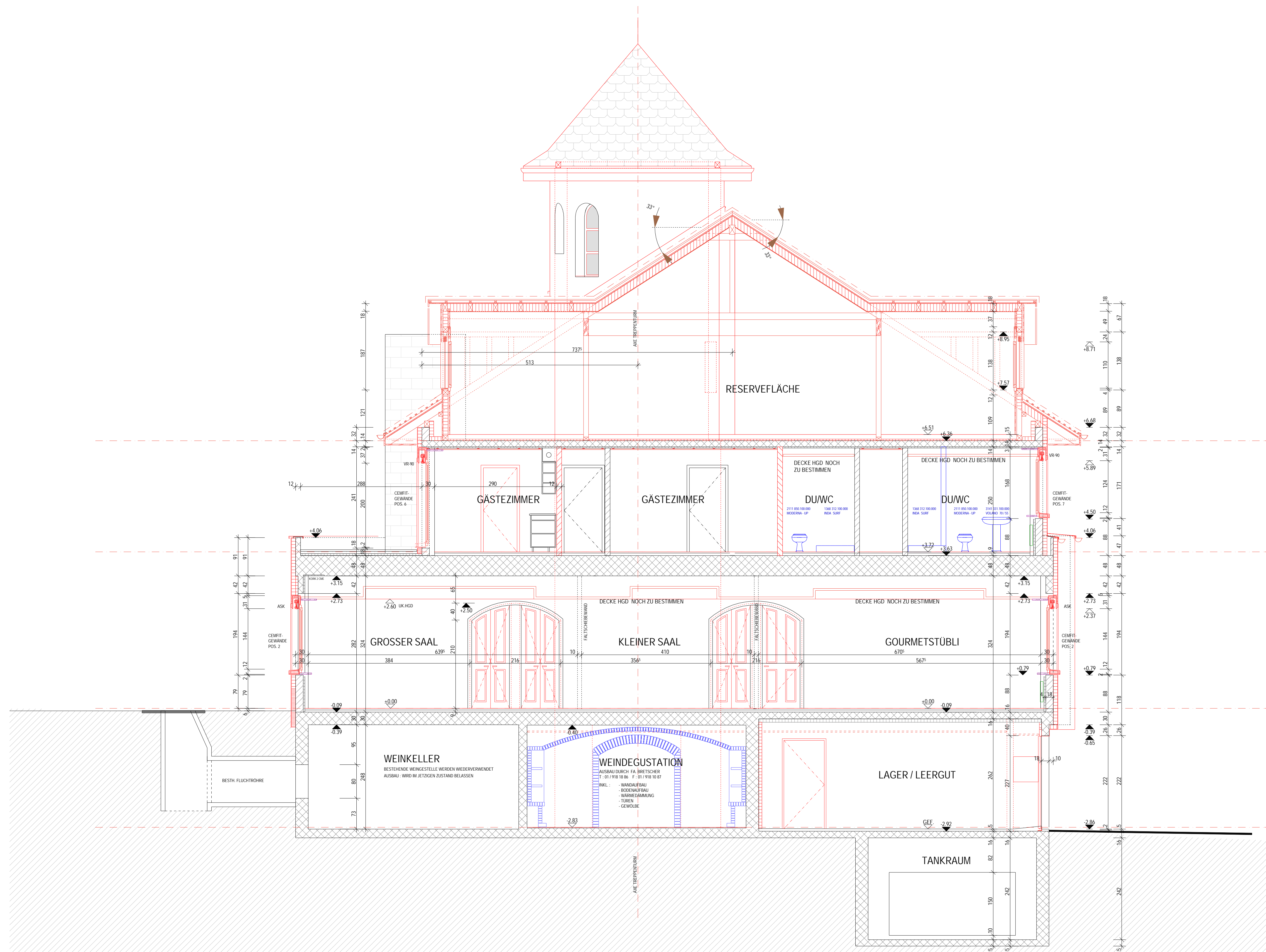
SCHNITT C-C
