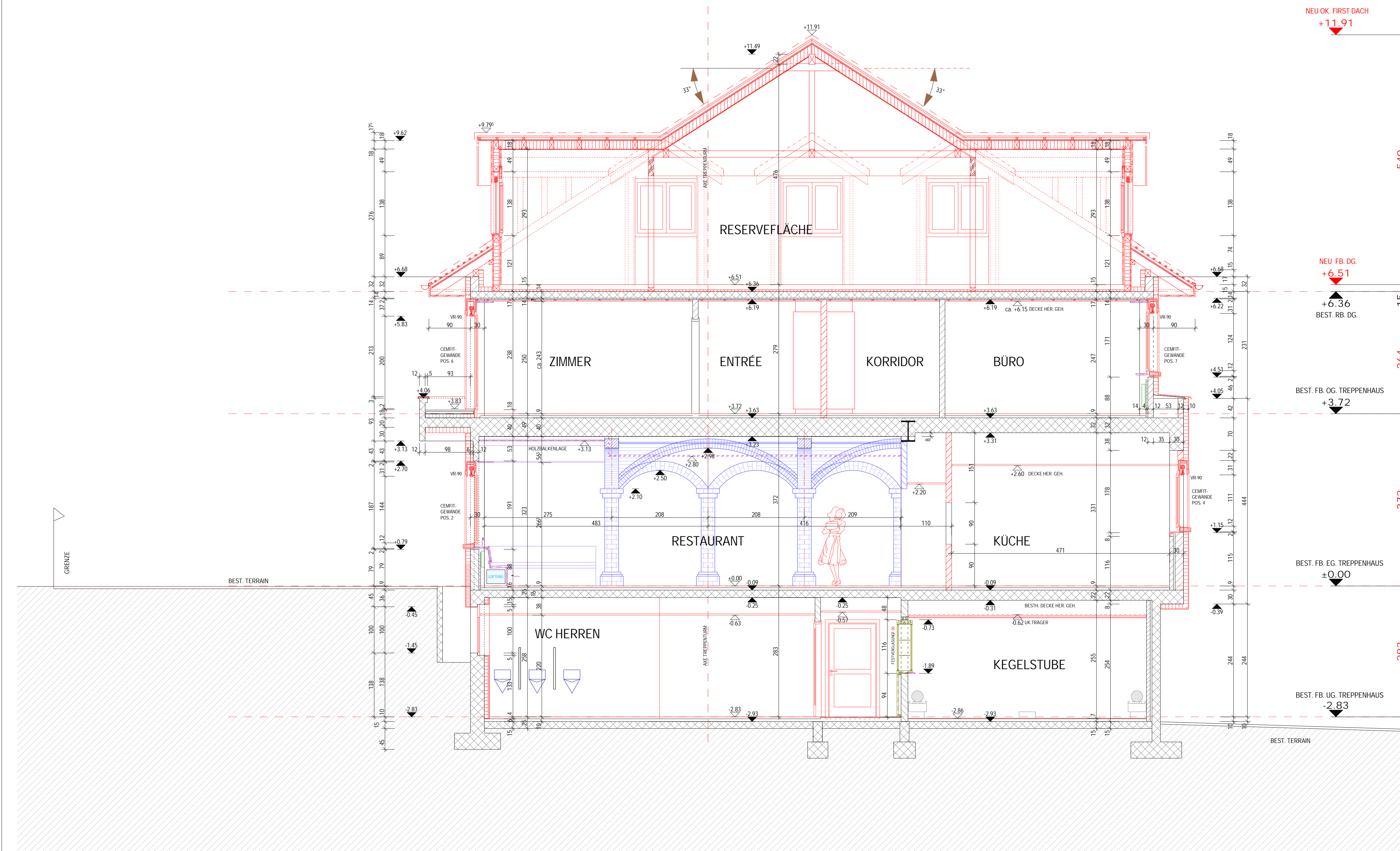
SCHNITT A-A
