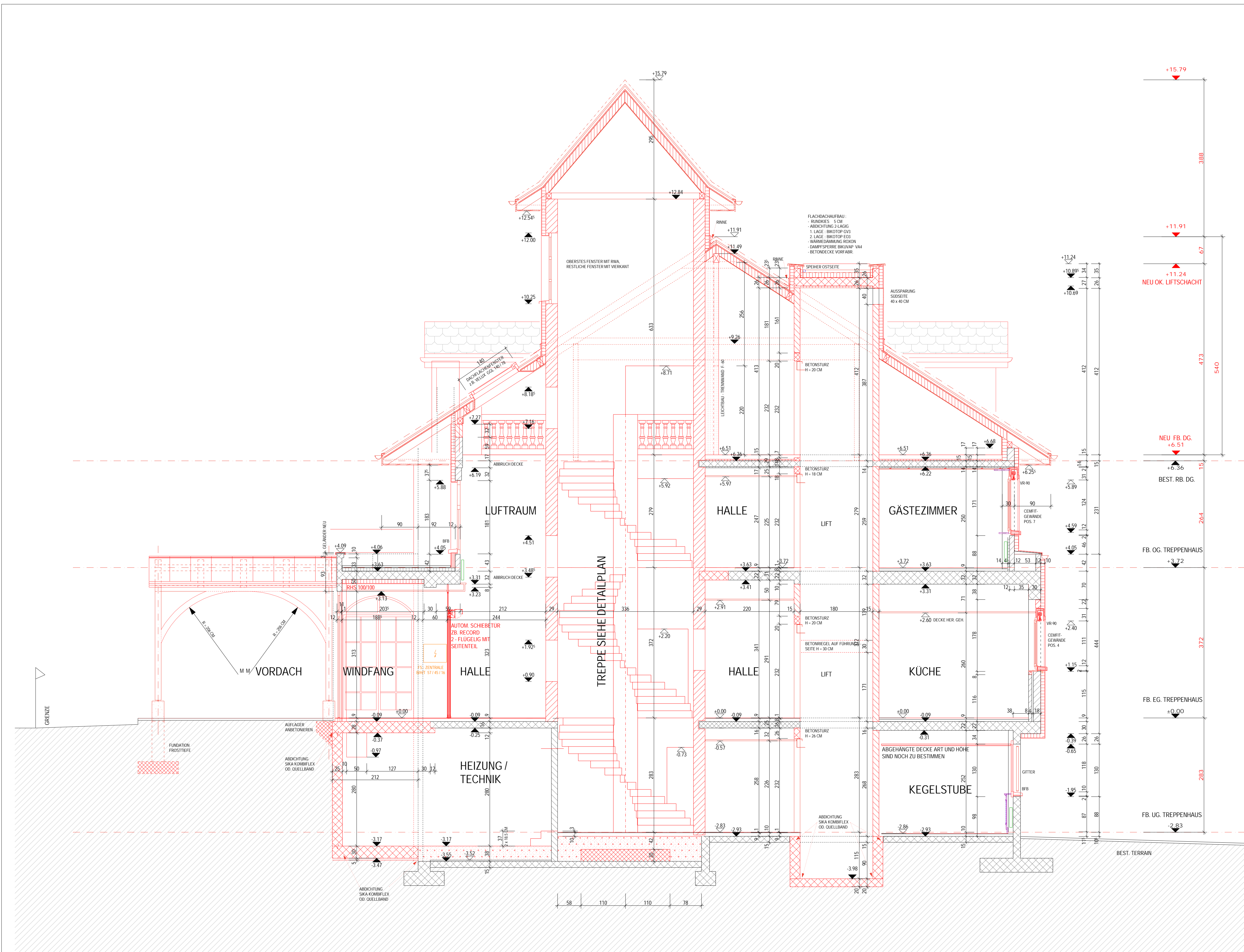
SCHNITT B-B
