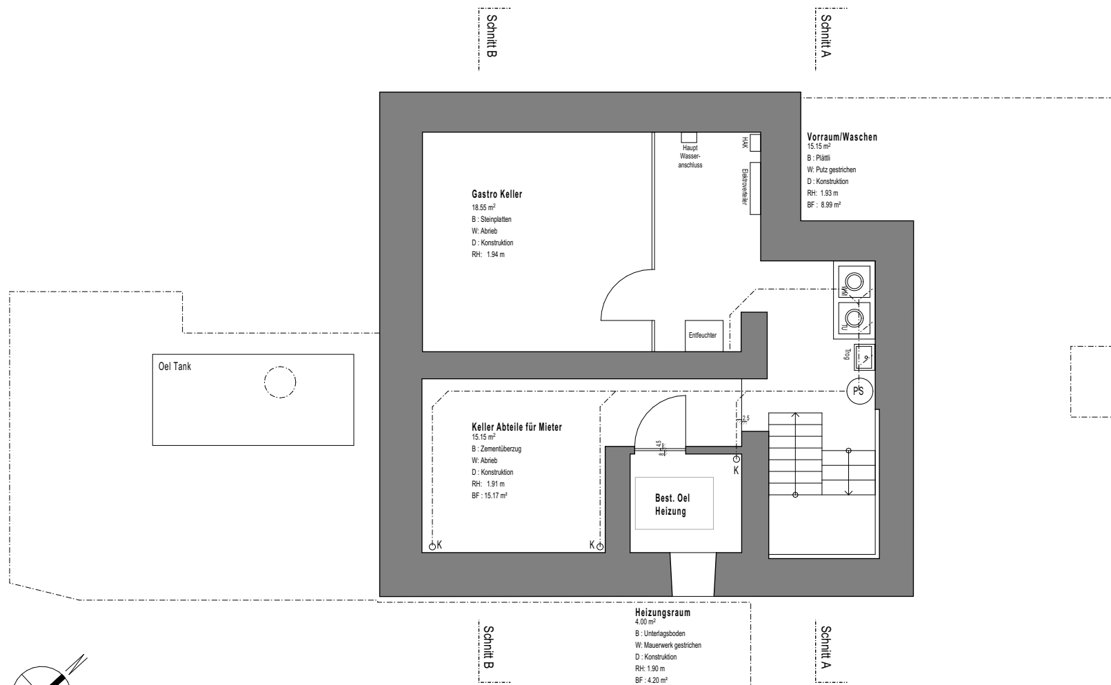
Grundriss UG
